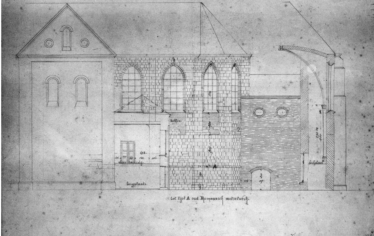
Zuidelyk aanzicht van het priesterkoor te Rolduc. Schaal 1 op 100
