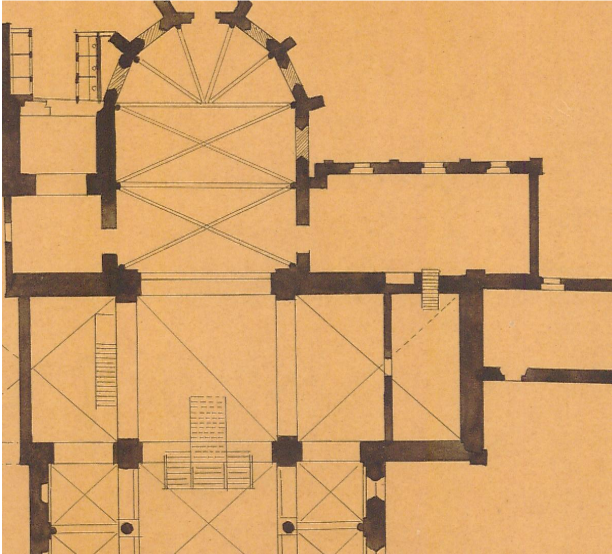
[de trap , 95 cm breed, [uit eigen schatting tekening cuypers] begint circa 1,25 meter vanaf de zuidwand; let op dat schildering maria horizontaal verdwijnt en links vertikaal]
